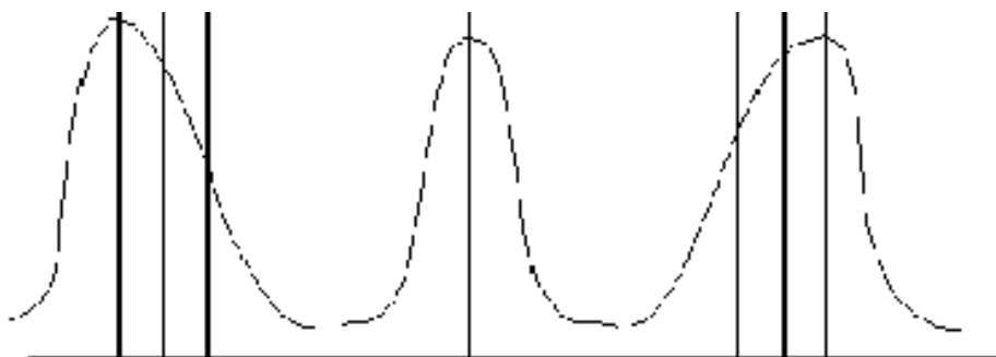
Рис.5.1. Типы кривых распределения (по асимметрии)
