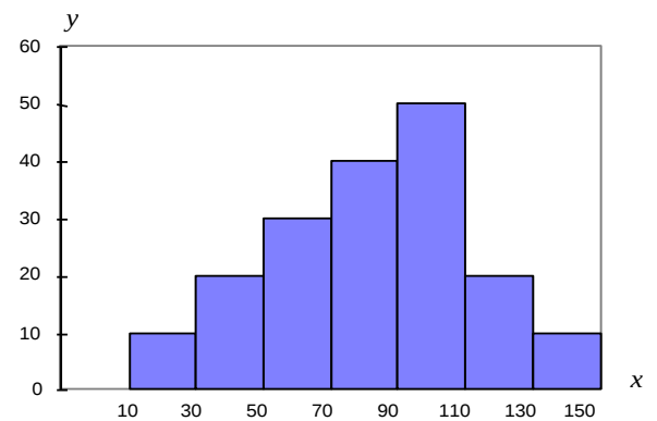
Рис. 2.3. Гистограмма распределения электродвигателей по мощности.
