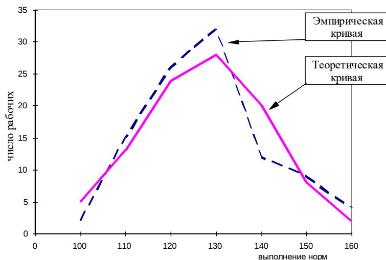
Рис. 5.3. Эмпирическое и теоретическое распределение рабочих по степени выполнения норм
