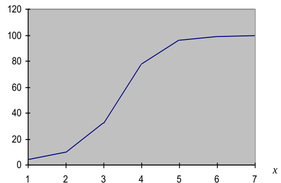
Рис. 2.2. Кумулята распределения квартир по числу проживающих в них лиц.
