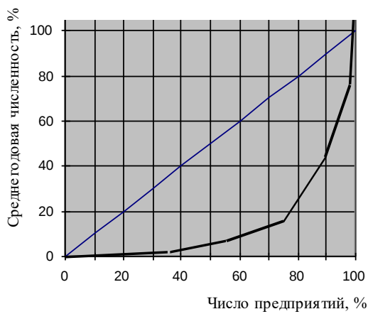
Рис. 2.4. График Лоренца
