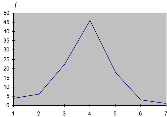
Рис. 2.1. Полигон распределения квартир по числу проживающих в них лиц
